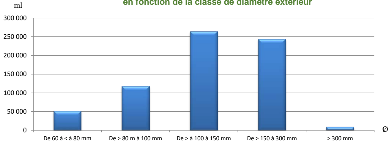
Figure 1 : Répartition des linéaires, pour les conduites considérées principales, en fonction de la classe de diamètre extérieur
