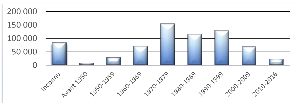
Figure 3 : Répartition des linéaires de réseaux en fonction l'âge des conduites principales
